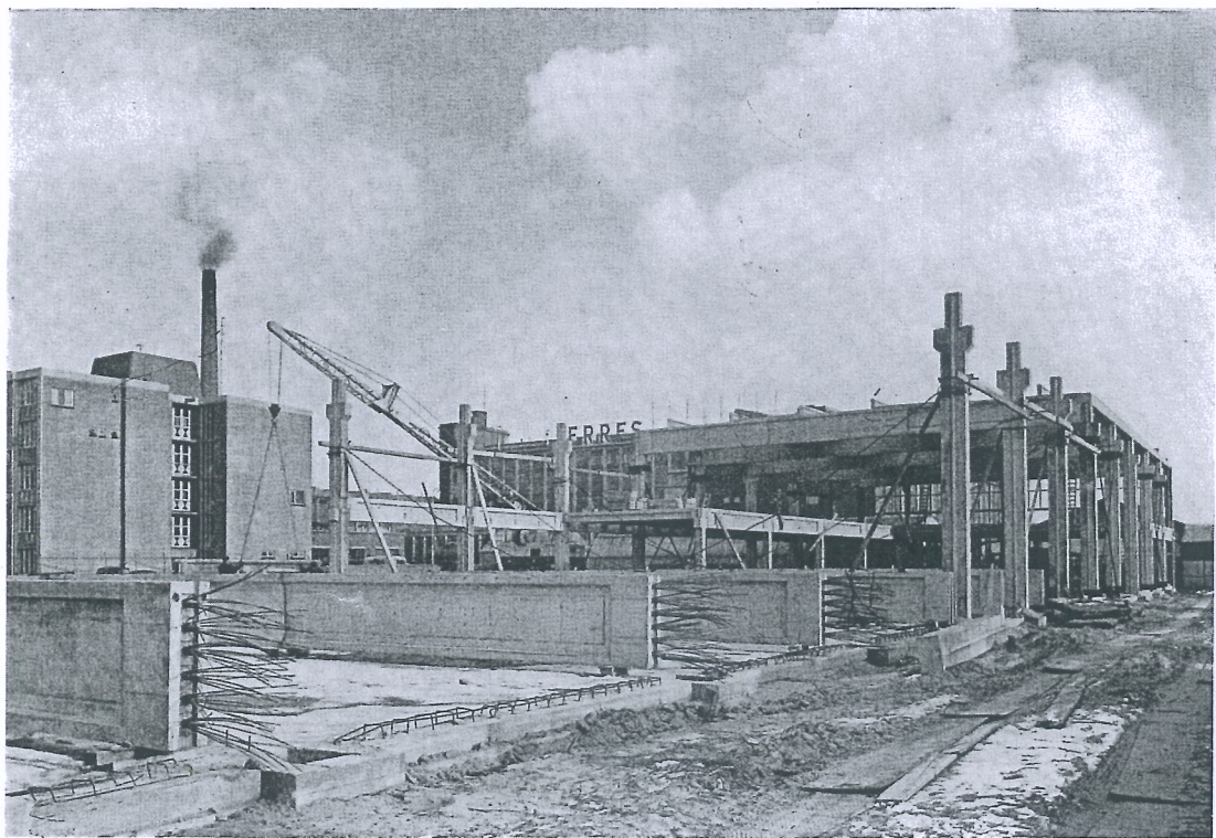
Boven: telecommunicatiegebouw en personeelsgebouw. Onder: uitbreiding. Van der Heem N.V. te Den Haag.
